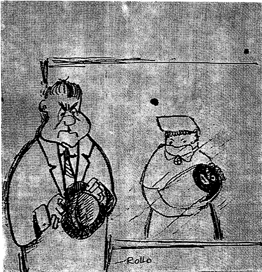
— Kiroitut ydinpommikokeet.
